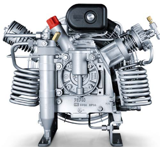
Компрессорный блок IK 120 (используется на PE-TE, HE, MVE и VE)
