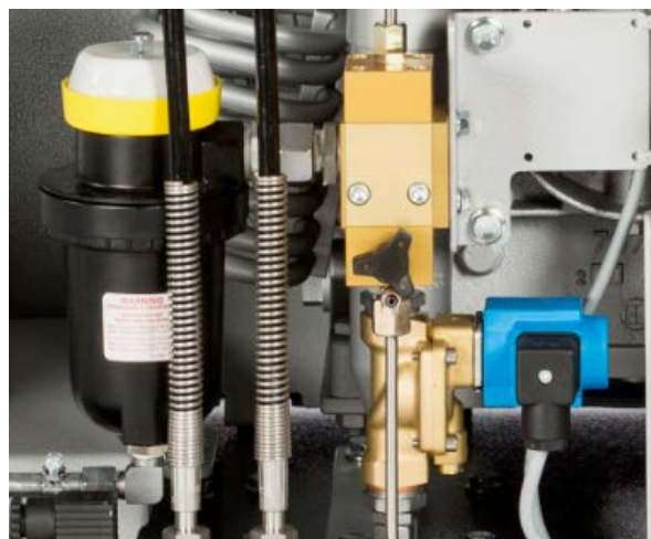
Автоматическая работа компрессора экономит время: система автоматического спуска конденсата, установленная на PE-TE
